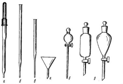
Рис. 1.4. Пипетки: а, б – каменные, в – для отделения жидкости от осадка Рис. 1.5. Химическая (а), капельная (б) и делительная (в) воронки
